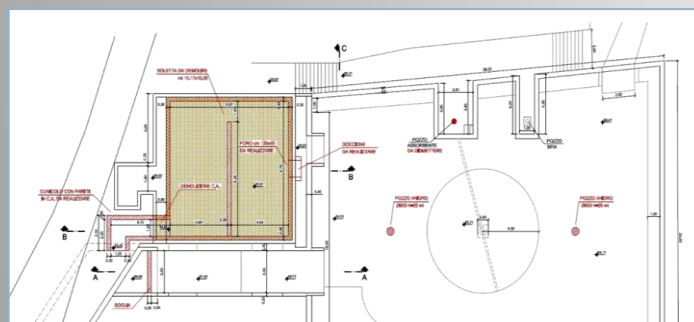
RECAPITO FINALE CIOLO
