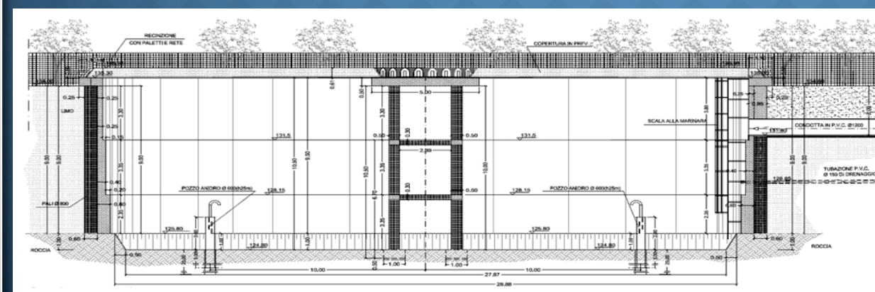
SEZIONE RECAPITO FINALE IN LOCALITÀ CUPONE
