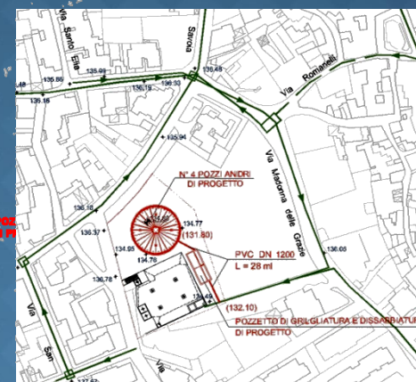
RECAPITO FINALE IN LOCALITÀ CUPONE
