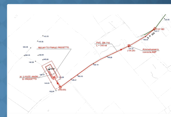
RECAPITO A SERVIZIO DELLA FRAZIONE DI S. DANA
